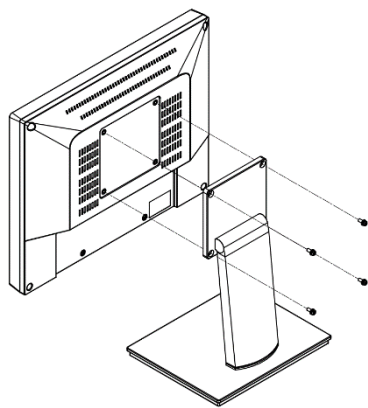
取付け図
